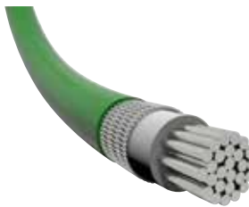
Kern: 26 geleiders
